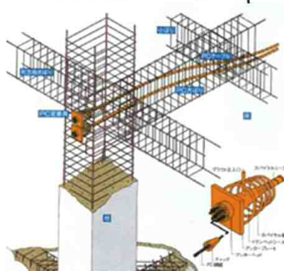
PC緊張
